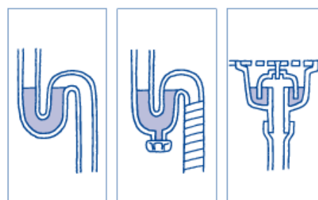
U字型排水トラップ
